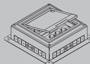
doza ETD-6M art. št: 441400 (RAL 9006) art. št: 441400RF (INOX)
