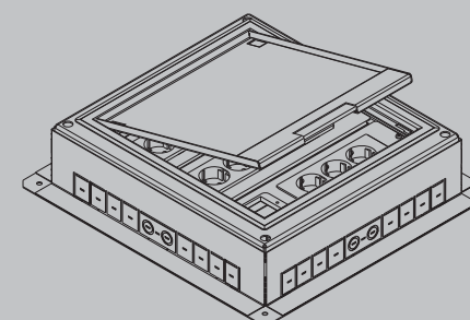
doza ETD-12M art. št: 443500 (RAL 9006) art. št: 443500RF (INOX)
