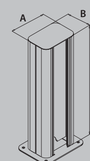
dvostranski stebriček AT-OK 160/110/500
