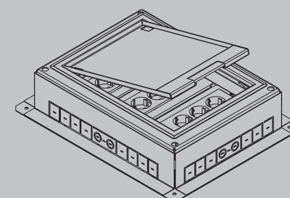
doza ETD-9M art. št: 442500 (RAL 9006) art. št: 442500RF (INOX)
